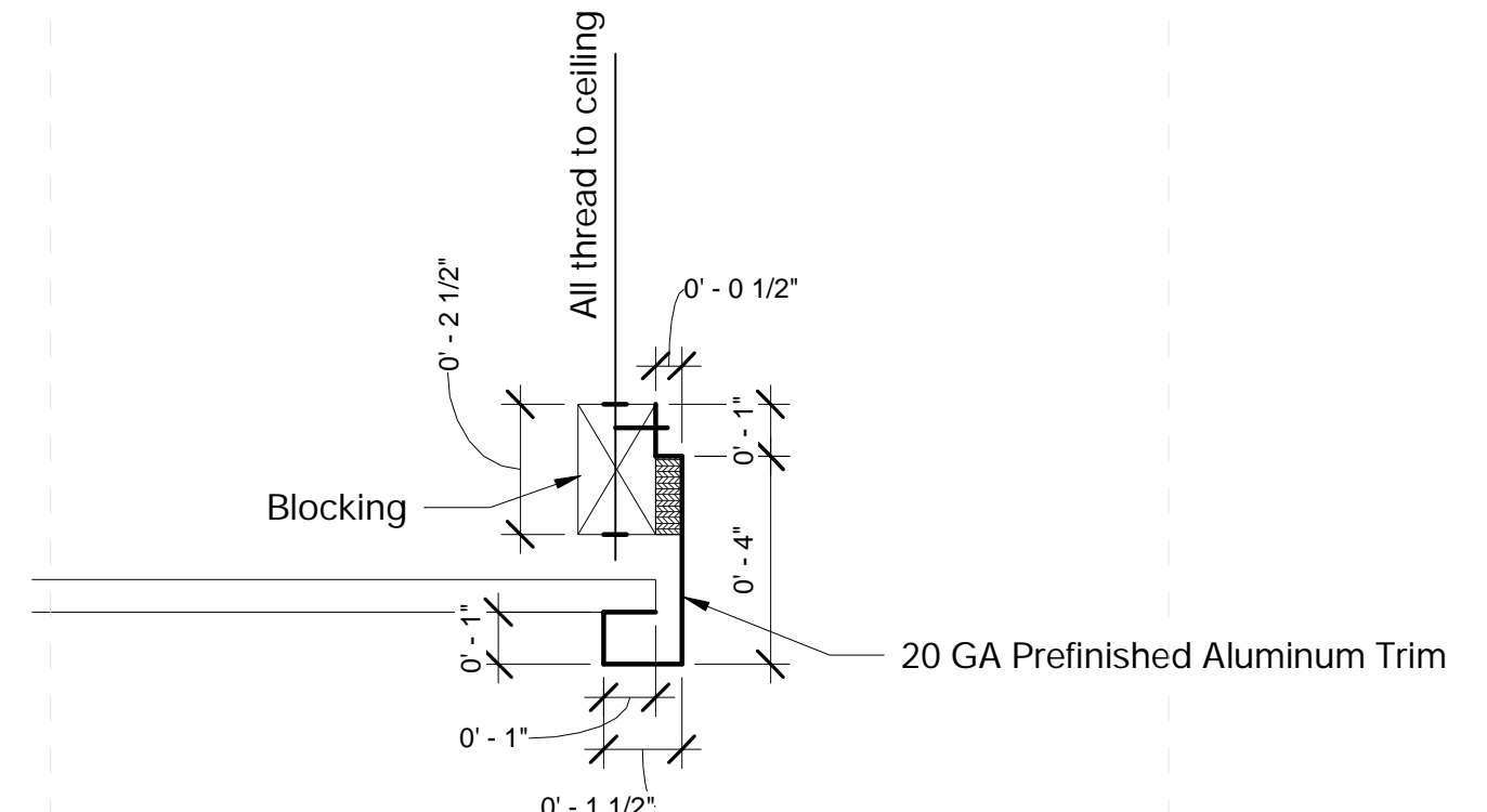
Ceiling Edge Trim Detail 3" = 1'-0"
